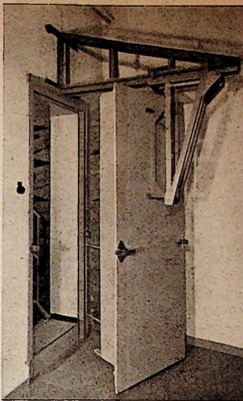
Fig. 4. De wegschuivende deur. Zie de ontworpen constructie aan de bovenzijde
