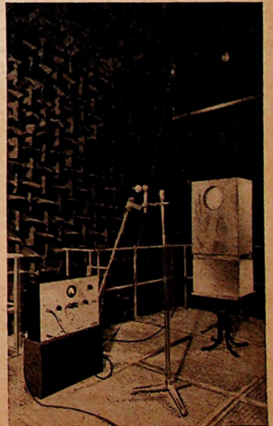
Fig. 3. De opstelling van de apparatuur op het rooster.
